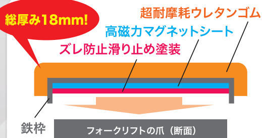
フレコン専用タイプ断面構造
