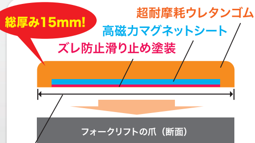
フレコン&パレット 兼用タイプ断面構造
